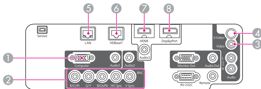
Input Port
